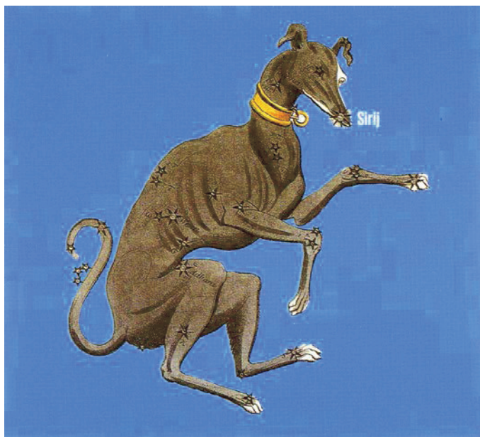
Legla zvezde Sirij v ozvezdju Veliki pes.
